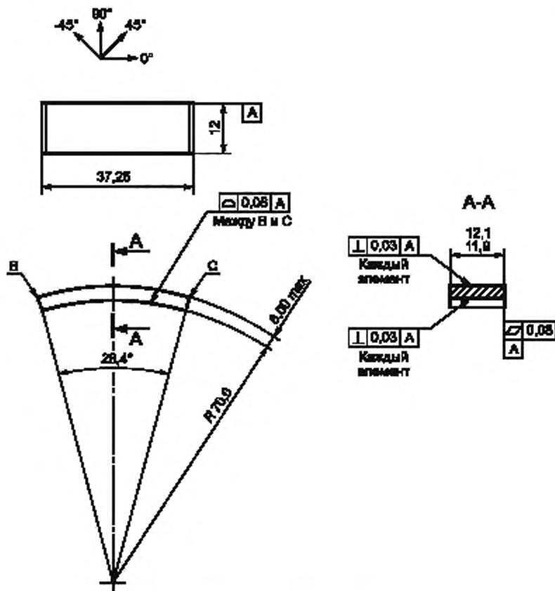
Рисунок 2 — Изогнутый образец
