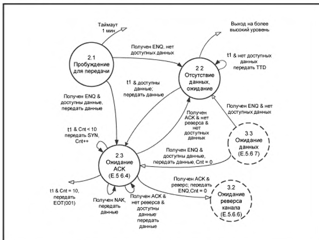
Рисунок Е.3 — Диаграмма перехода состояний передатчика
