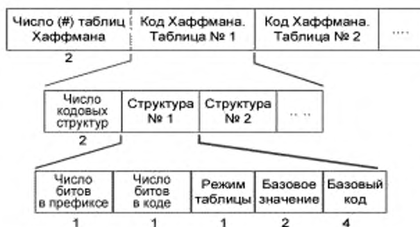
Рисунок 5 — Обзор структуры раздела таблиц Хаффмана
