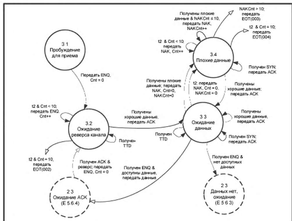
Рисунок Е.6 — Диаграмма перехода состояний приемника
