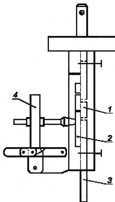
1 — образец; 2 — адаптер; 3 — нагружающее приспособление; 4 — фиксатор
