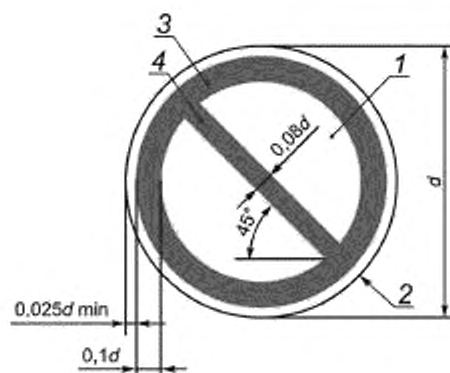
Рисунок А.1 — Основа цветового изображения и соотношение размеров запрещающих знаков безопасности
