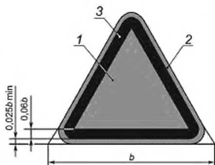
b — сторона треугольника; 1 — основная поверхность; 2 — кант; 3 — кайма
