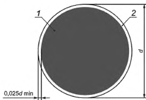
d — диаметр круга; 1 — основная поверхность; 2 — кант
