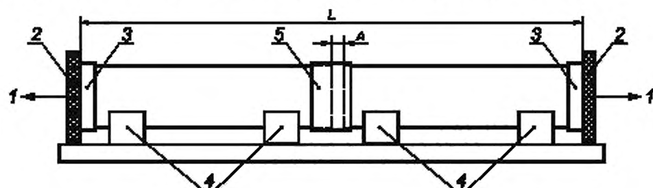
1 — осевое давление, действующее на образец для испытаний; 2 — оснастка испытательного стенда; 3 — торцевая заглушка; 4 — опоры; 5 — испытуемое соединение; A — общий вырыв; L — общая эффективная длина
