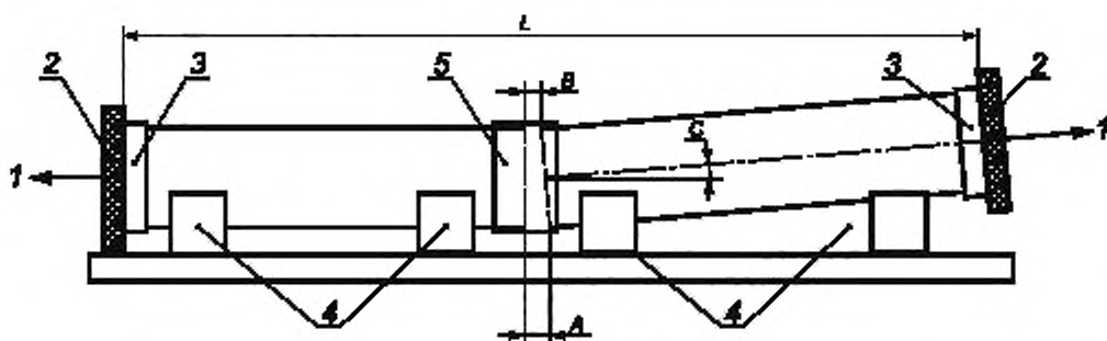
1 — осевое давление, действующее на образец для испытаний; 2 — оснастка испытательного стенда; 3 — торцевая заглушка; 4 — опоры; 5 — испытуемое соединение; A — общий вырыв; B — вырыв; C — угловое смещение; L — общая эффективная длина
