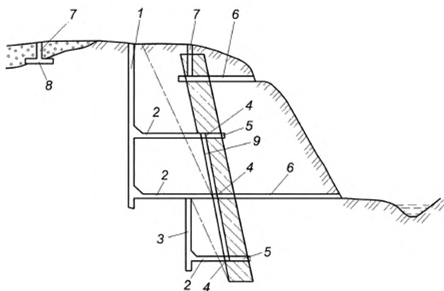
1 — ствол шахты; 2 — квершлага; 3 — слепой ствол; 4 — штреки; 5 — орты; 6 — штольни; 7 — шурфы. 8 — рассечка; 9 — восстающий
