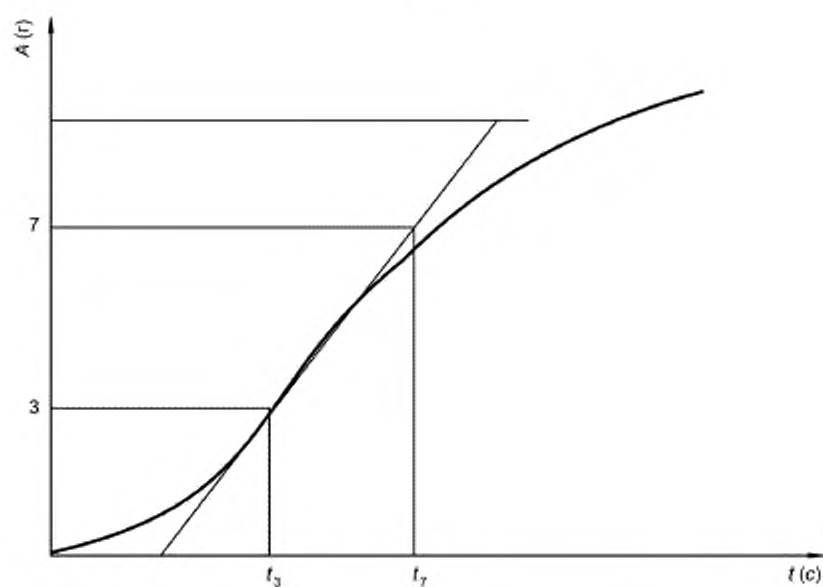
Рисунок А.2 — Калибровка пористой среды
