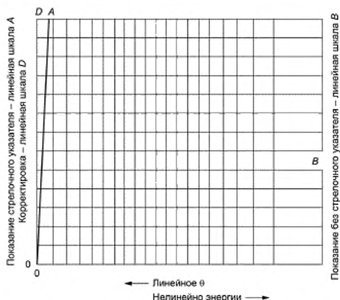
Рисунок А1.2 — Образец диаграммы корректировки сопротивления ветра и трения \theta
