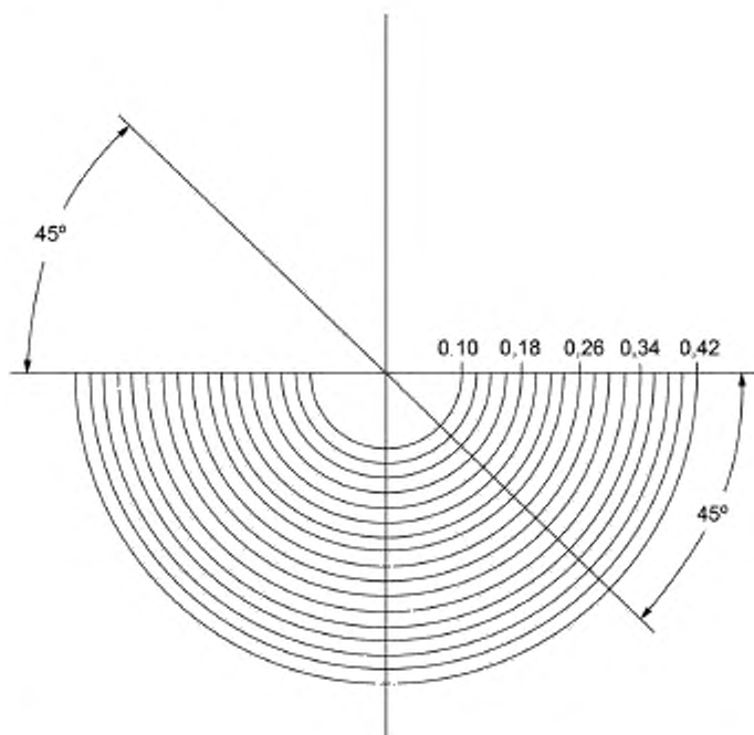
Рисунок А.1 — Пример прозрачного шаблона для увеличения 100х
