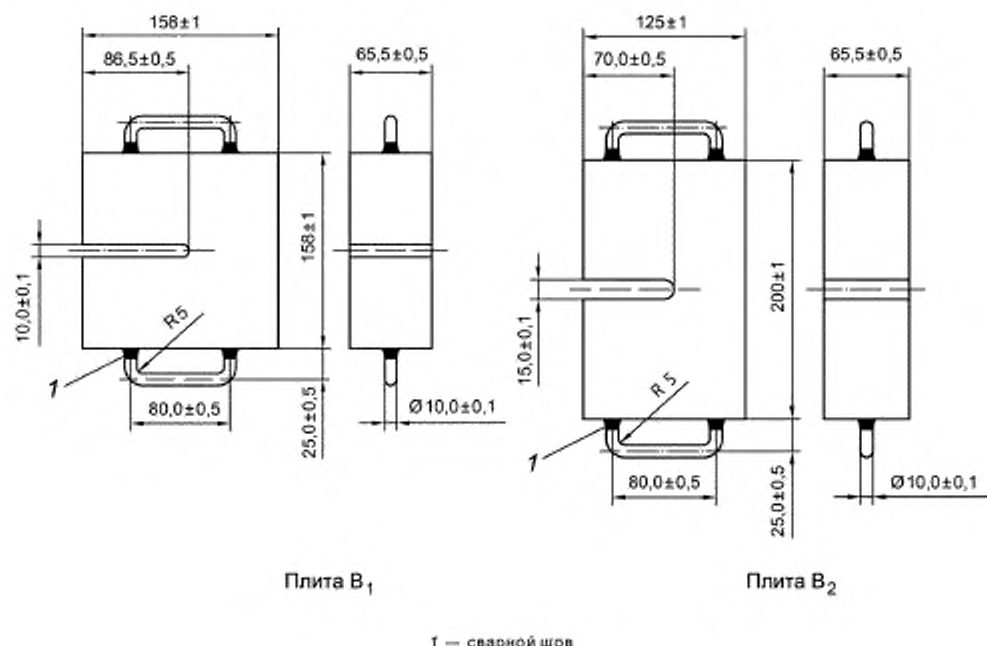
Рисунок 3 — Геометрические размеры плиты В
