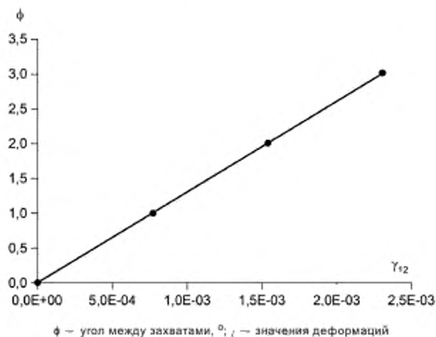
Рисунок 5 — График дефекта кручения
