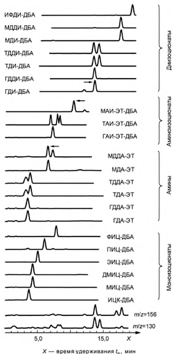
Рисунок В.1 — ЖХ-МС хроматограмма раствора, содержащего 0,15 мкг/см 3 различных ДБА-производных изоцианатов, ЭХФ-ДБА-производных аминизоцианатов и ЭХФ-производных аминов
