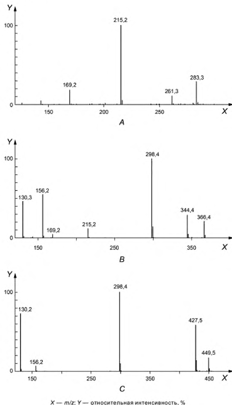
Рисунок В.4 — Масс-спектры с указанием относительной интенсивности для ЭТ-производного ГДА (А), ЭХФ-ДБА-производного ГАИ (В) и ДБА-производного ГДИ (С), полученные методом жидкостной хромато-масс-спектрометрии (ЖХ-МС) с обращенной фазой с электрораспылительной ионизацией (ЭРИ)
