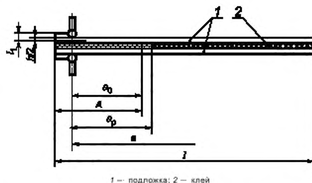
Рисунок 2 — Образец для испытания методом ДКБ с петлями (альтернативный режим нагружения)
