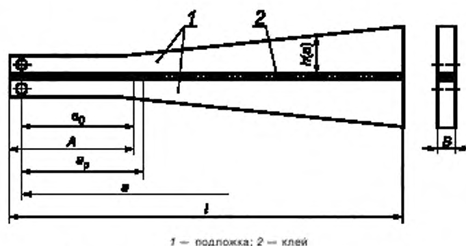
Рисунок 4 — Образец для испытания методом КДКБ
