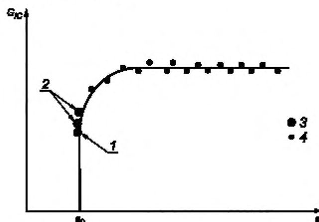
1 — самая низкая точка страгивания (наименьшее значение среди НЛ, ВИЗ и МАХ/5%); 2 — другие точки страгивания; 3 — значения страгивания; 4 — значения распространения
