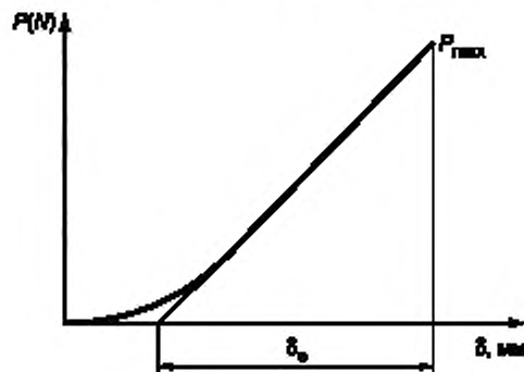
Рисунок A.1 — Схематическая картина зависимости «нагрузка — смещение», полученная в процессе измерения податливости системы
