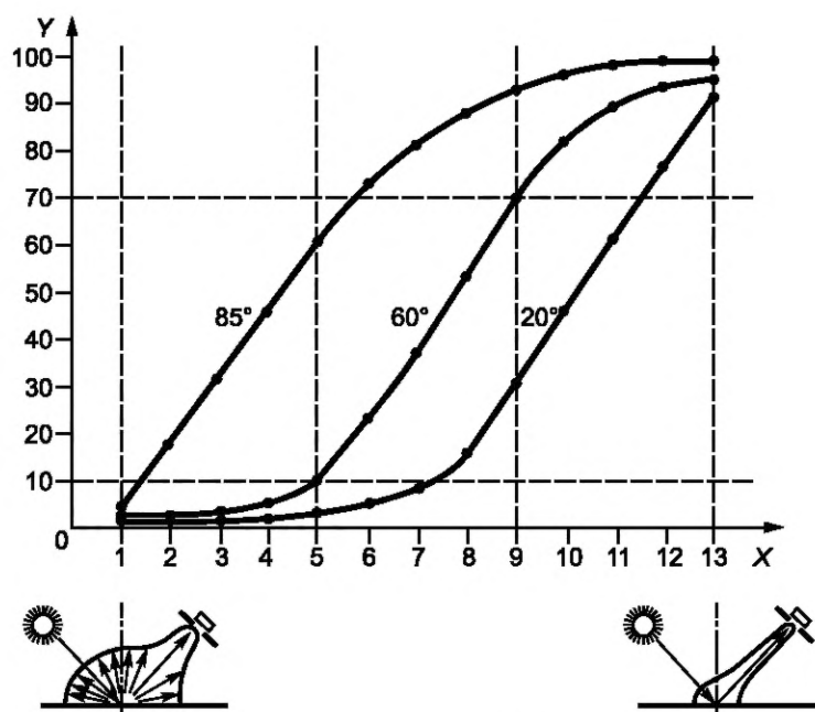
Рисунок 1 — Кривые блеска
