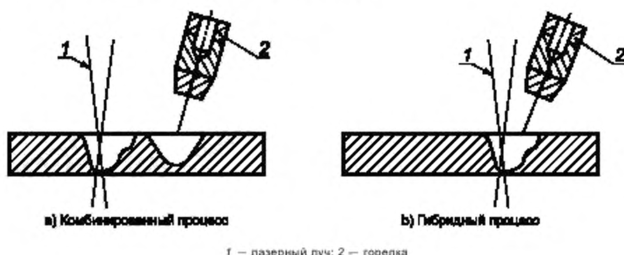
Рисунок 1 — Комбинация сварочных процессов
