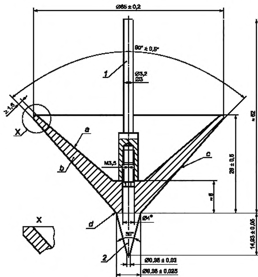
1 — падающий стержень из нержавеющей стали; 2 — наконечник иглы (из закаленной упроченной или нержавеющей стали); a — обрабатывают до требуемой массы; b — латунь или коррозионно-стойкая сталь; c — гладкая, полированная поверхность; d — плотная посадка, e — плавный переход без выступа
