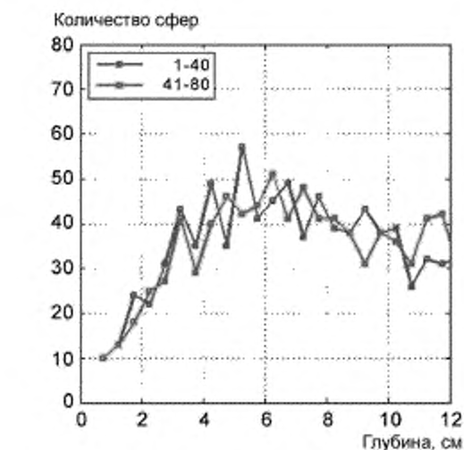
б Число центров слабоотражающих сфер, выявленных в каждом пятимиллиметровом интервале глубины
