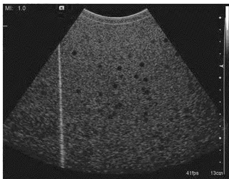
Рисунок В.1 — Изображение образца фантома со слаботражающими сферами диаметром 4 мм для использования в диапазоне частот от 2 до 7 МГц, полученное с помощью датчика с конвексной решеткой
