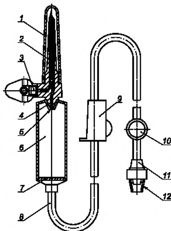
1 — защитный колпачок иглы для прокола крышки емкости; 2 — игла для прокола крышки емкости; 3 — воздуховод с воздушным фильтром и заглушкой; 4 — жидкостной канал; 5 — каплеобразующий элемент; 6 — капельная камера; 7 — жидкостной фильтр; 8 — трубка; 9 — роликовый зажим; 10 — инъекционный узел; 11 — головка с конусом «Луер»; 12 — защитный колпачок на головку с конусом
