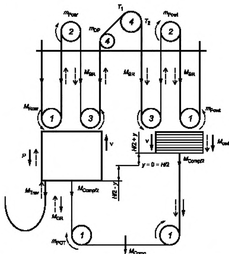
1, 2, 3, 4 — фактор линейной скорости вращения блоков, например 2 = 2 \cdot v_{car} ; H — высота подъема, м; M_{CR} — расчетная масса компенсирующих канатов или цепей ( [0,5 H \pm y] ); n_c — масса компенсирующего каната/цепи на единицу длины, кг; y — на уровне 0,5 H \pm y = 0 , м; n_c — количество компенсирующих канатов/цепей; M_{CR} — расчетная масса тяговых канатов ( [0,5 H \pm y] ); n_s — масса каната на единицу длины, кг; n_s — количество тяговых канатов; \rightarrow направление статической силы; \cdots — направление динамической силы
