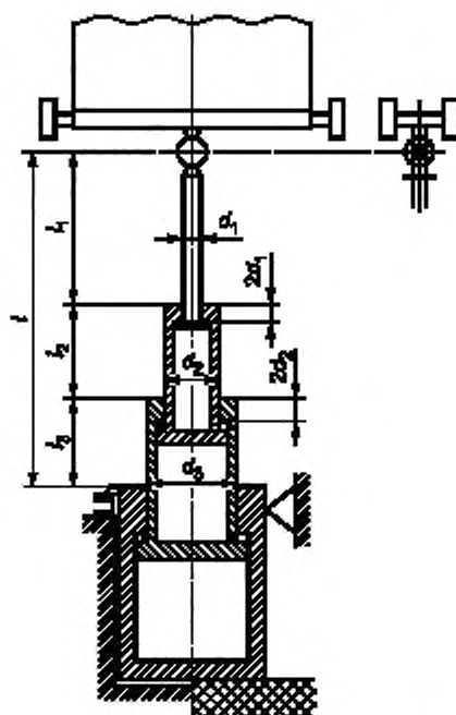
Рисунок 12 — Телескопические гидроцилиндры без внешней направляющей
