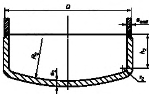
Рисунок 9 — Выгнутое основание
