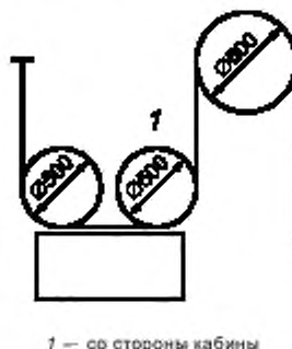
Рисунок С.1 — Полиспастная подвеска 2:1. Канатоведущий шкив с клиновой канавкой
