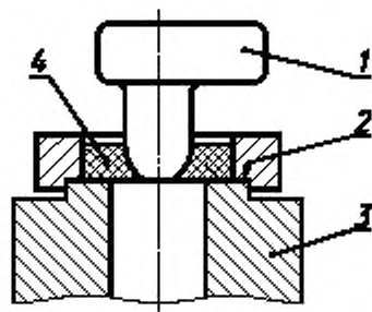
Рисунок 4 — Соединение слухового аппарата типа «ушная вставка» (изготовленного по заказу) с имитатором закрытого уха
