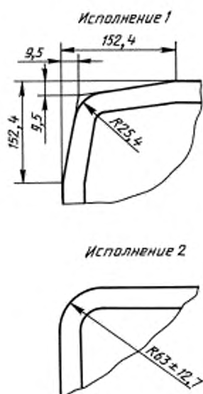
Рисунок 5 — Размеры основания (вид сверху)
