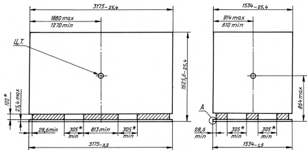
Рисунок 2 — Прямоугольный контейнер (контейнер типоразмера 2)
