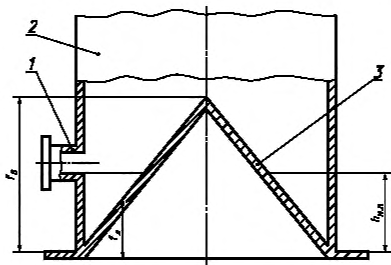
1 — приемно-раздаточный патрубок; 2 — стенка резервуара; 3 — неровности днища; f_{\delta} — высота неровностей днища; f_{\Delta} — высота точки касания днища грузом рулетки; h_{м.п.} — высота «мертвой» полости
