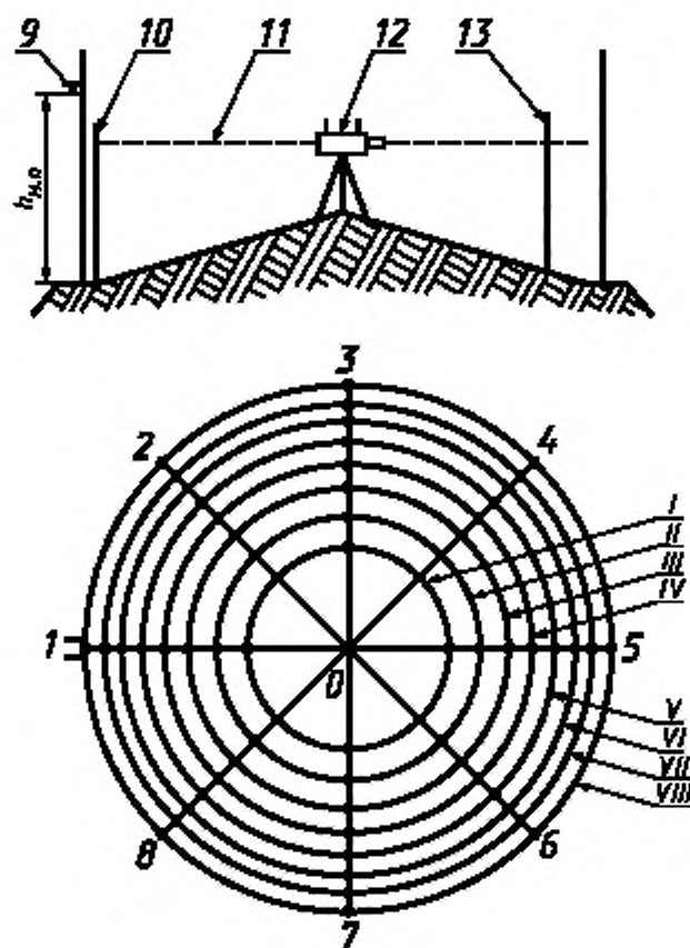
1—8 — радиусы, 9 — приемно-раздаточный патрубок; 10 — рейка; 11 — горизонт нивелира; 12 — нивелир; 13 — рейка в точке касания дна грузом рулетки; I—VIII — концентрические окружности; h_{м.д.} — высота «мертвой» полости резервуара
