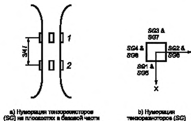
Рисунок В.1 — Установка тензодатчиков на поверхности в базовой части и их нумерация
