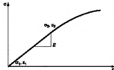
Рисунок 1 — Механические характеристики с линейным участком, который ограничен \sigma_1, \varepsilon_1 и \sigma_2, \varepsilon_2
