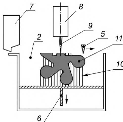
б) Электронно-лучевое сплавление материала в сформированном слое
