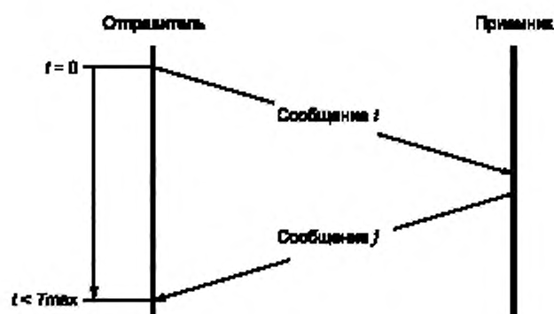
Рисунок 3 — Двухнаправленная передача сообщений
