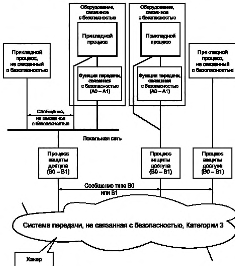
Рисунок С.7 — Коммуникация между связанными и не связанными с безопасностью приложениями
