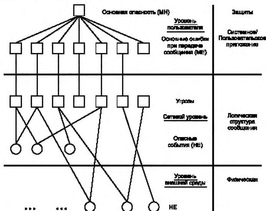
Рисунок А.1 — Дерево опасности
