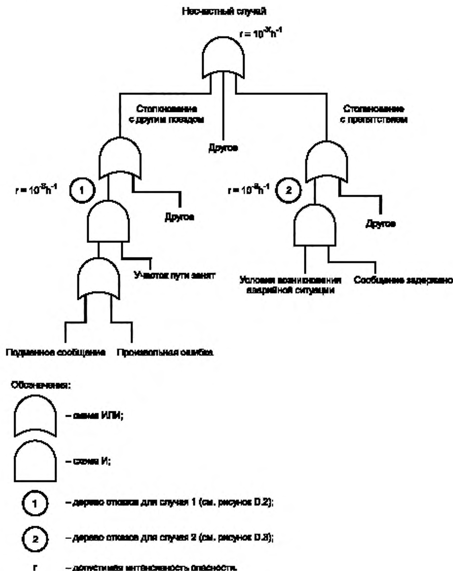
Рисунок D.1 — Дерево отказов для опасности «авария»
