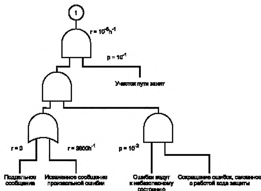
Рисунок D.2 — Дерево отказов для случая 1
