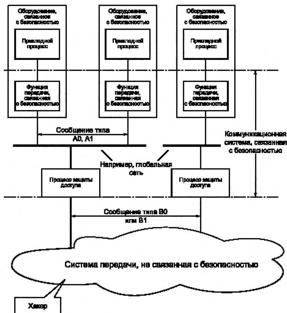
Рисунок С.3 — Использование отдельного слоя защиты доступа
