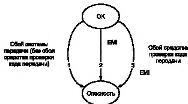
Рисунок С.6 — Базовая модель ошибки
