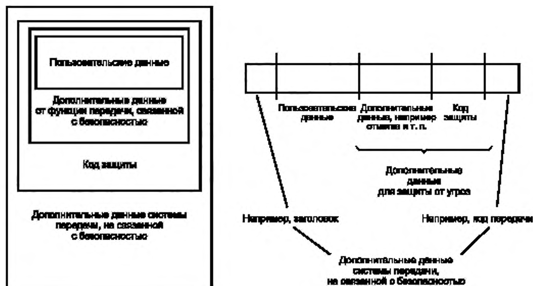
Рисунок С.2 — Модель представления сообщения в системе передачи (тип A0, A1)
