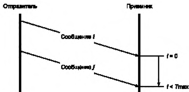
Рисунок 2 — Циклическая передача сообщений
