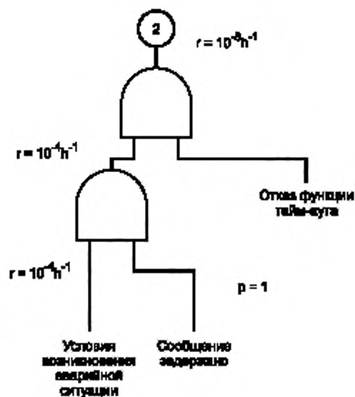
Рисунок D.3 — Дерево отказов для случая 2
