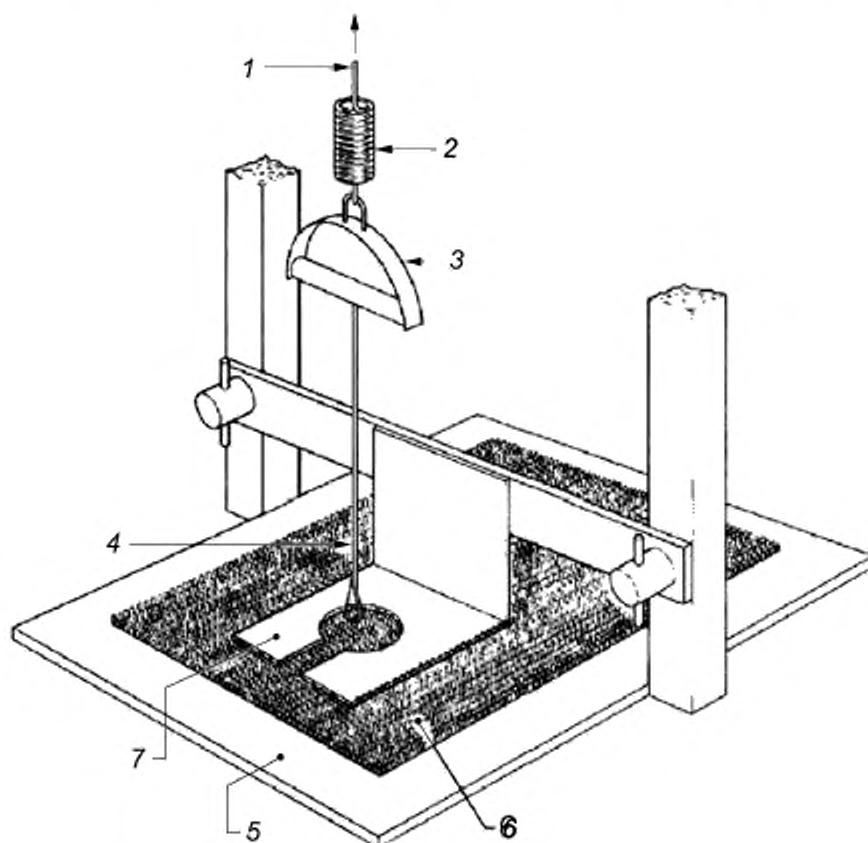
1 — нагружающий механизм, 2 — пружина (если необходимо); 3 — верхний захват; 4 — захват для пучка или крючок для петли; 5 — опорная плита; 6 — образец ковра; 7 — зажим для образца, размеры по 5.1
