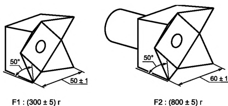
Рисунок 2 — Испытательный снаряд
