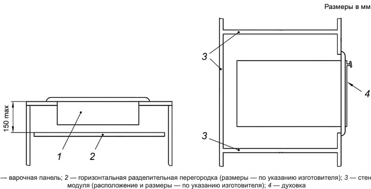
Рисунок 4 — Пример испытательного модуля для встраиваемых приборов класса 3
