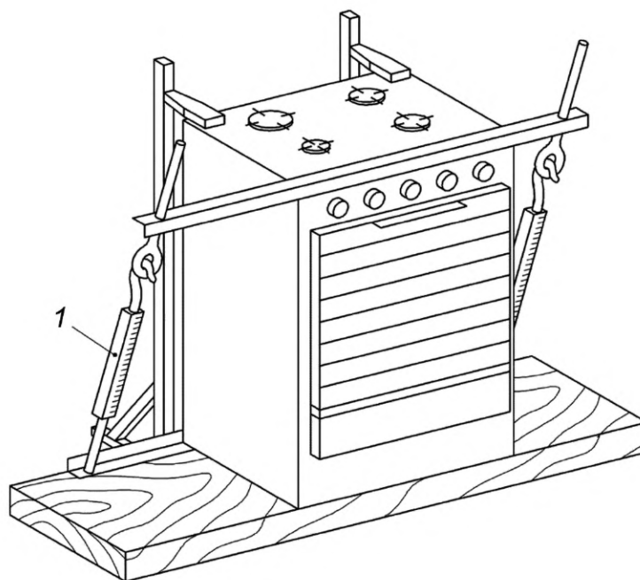
1 — динамометр
