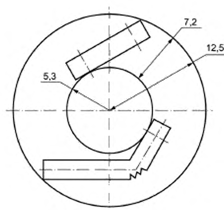
Рисунок 1 — Схема поворота транспортного средства
