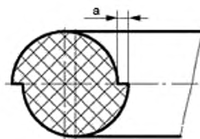
Рисунок 5 — Смещение a
