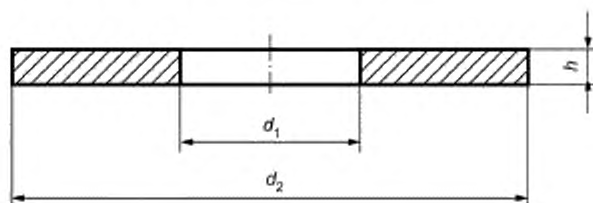
Рисунок 1 — Размеры
