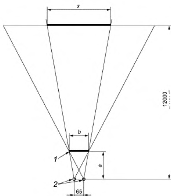
1 — конструктивный элемент, препятствующий обзору; 2 — глаза; a — расстояние между конструктивным элементом, препятствующим обзору, и точкой расположения глаз оператора; b — ширина конструктивного элемента, препятствующего обзору; x — зона затенения
