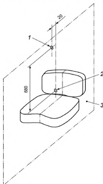
1 — центральная точка вращающейся опоры (FCRP); 2 — контрольная точка сиденья (SIP); 3 — плоскость, параллельная продольной плоскости трактора
