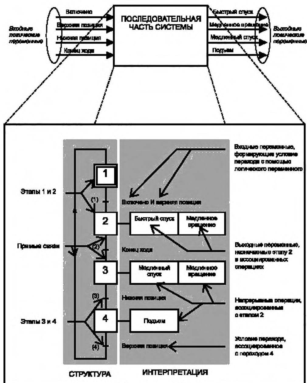
Рисунок 2 — Элементы структуры и интерпретации, используемые в диаграмме grafcet для описания поведения последовательной части системы, определяемой ее входными и выходными переменными
