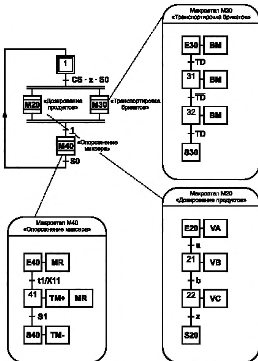
Рисунок В.4 — Диаграмма grafset устройства взвешивания-смешивания с использованием глобального описания на основе макроблоков и детального описания с помощью расширений макроблока
