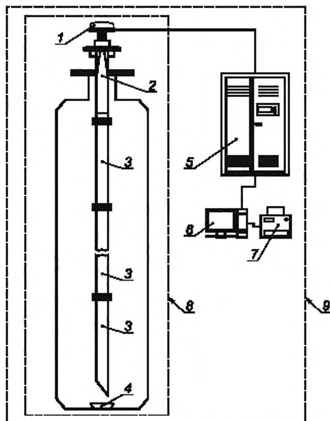
1 — микроволновый передатчик; 2 — антенна; 3 — стальная трубка; 4 — аттенюатор; 5 — управляющий блок; 6 — дисплейный блок; 7 — принтер; 8 — АРУ; 9 — система АРУ
