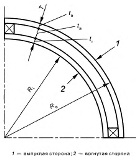
Рисунок 2 — Толщина и радиусы моллированного стеклопакета
