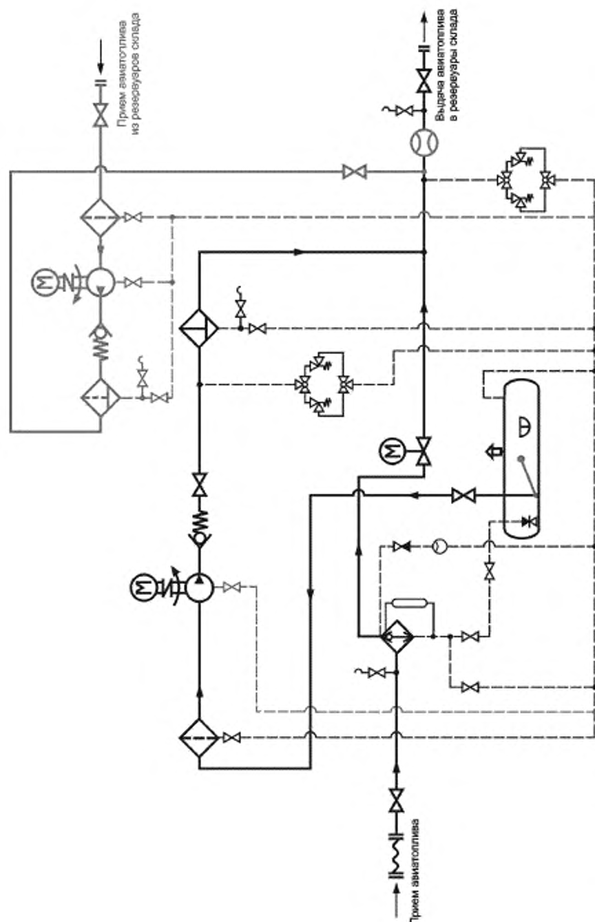
Рисунок Б.3 — Прием авиатоплива из танков нефтеналивных судов, стоящих на рейде, с гидроопорожнением шланговых устройств
