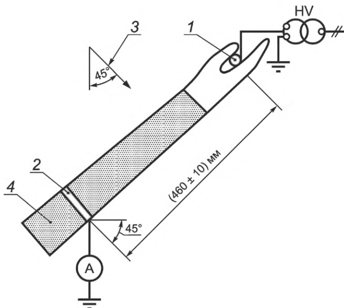
1 — голый электрод; 2 — электрод из проводящей изоляционной ленты; 3 — дождь; 4 — цилиндрическое удерживающее устройство; A — амперметр
