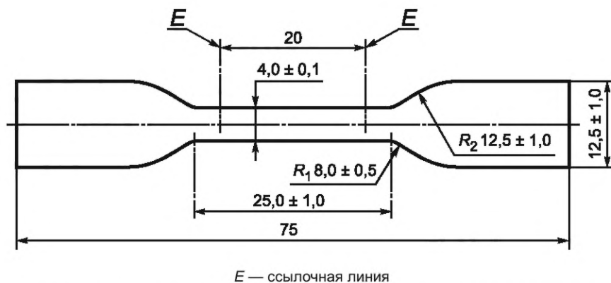
Рисунок 5 — Образец для испытаний на физико-механические показатели
