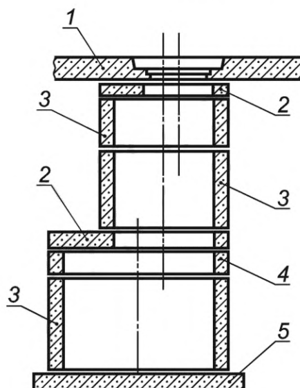
1 — плита перекрытия дорожная ПД; 2 — плита перекрытия ПП; 3 — кольцо стеновое цилиндрическое КС; 4 — кольцо опорное стеновое КО; 5 — плита дна ПН
