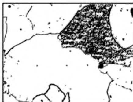
Балл 5, 500 х
