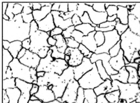
Балл 7, 500 х
