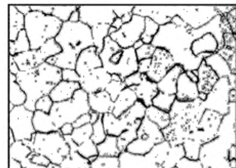
Балл 7, 500 \times , химическое травление
