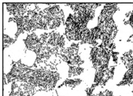
Балл 3, 100 х
