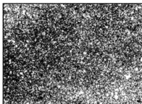
Балл 1, 100 \times , электролитическое травление
