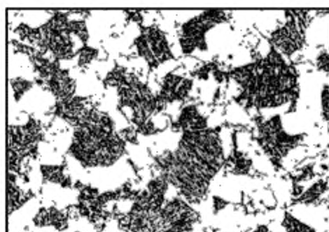
Балл 4, 100 х
