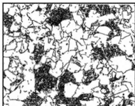
Балл 5, 100 х
