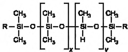
Рисунок 2 — Типичный полимерный сшивающий агент
