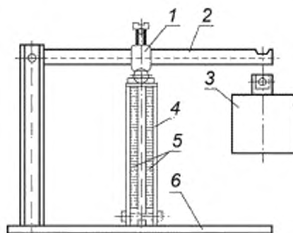
1 — движок; 2 — рычаг; 3 — груз; 4 — кассета; 5 — образцы; 6 — основание
