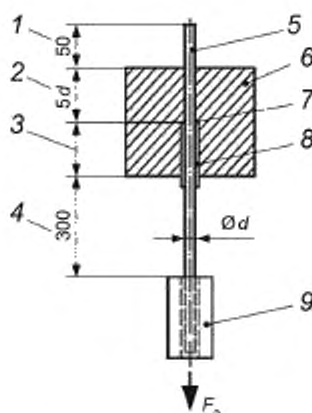
1 — часть стержня до точки применения устройства измерения смещения; 2 — длина сцепления; 3 — свободная преддлина 5d , миним. 200 мм \cdot 5d ; 4 — часть стержня до точки приложения силы растяжения; 5 — арматурный стержень; 6 — бетон; 7 — закупоривание; 8 — пластмассовая трубка; 9 — захват испытательной машины
