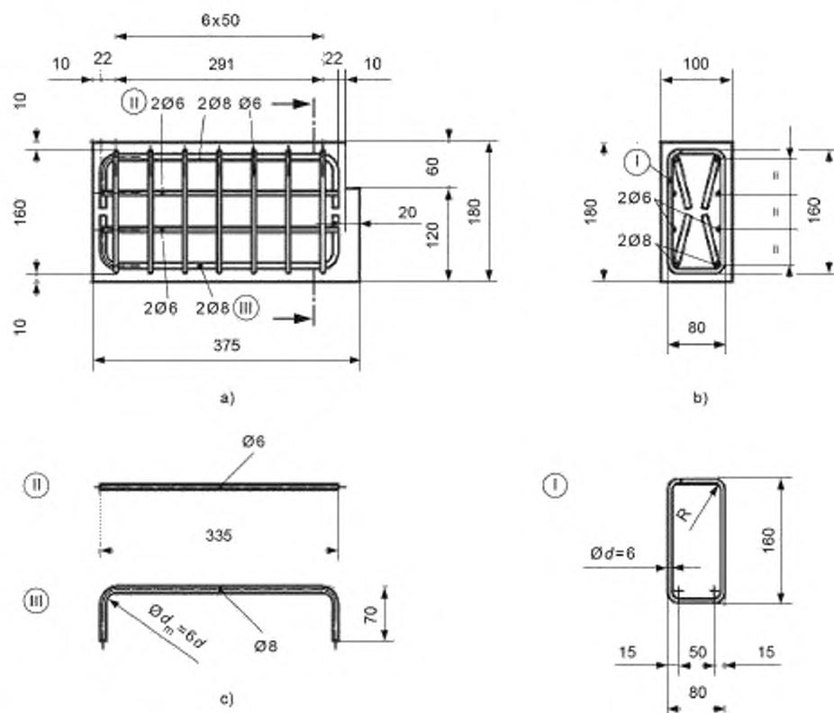
Рисунок С.5 — Балочное испытание типа А ( d < 16 мм). Арматура балочных образцов
