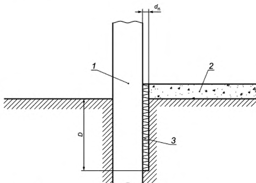
1 — стена фундамента; 2 — плита перекрытия на грунте; 3 — вертикальная изоляция; d_n — толщина изоляции фундамента; D — глубина вертикальной изоляции фундамента ниже уровня земли (грунтового основания)
