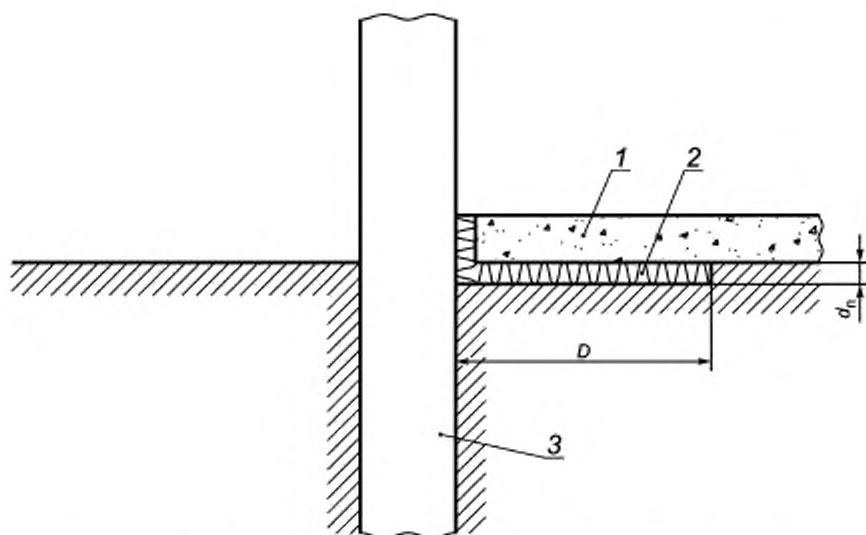
1 — плита перекрытия; 2 — горизонтальная изоляция; 3 — стена фундамента; d_{из} — толщина изоляции основания; D — ширина горизонтальной изоляции
