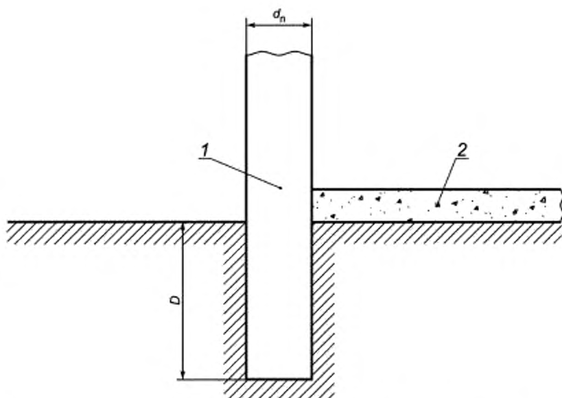
1 — стена фундамента низкой плотности \lambda_n < 1 ; 2 — плита перекрытия на грунте, d_n — толщина изоляции фундамента; D — глубина вертикальной изоляции фундамента ниже уровня земли (грунтового основания)
