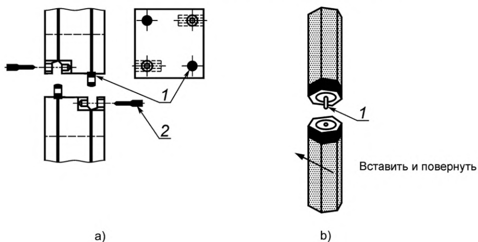
1 — установочный штифт; 2 — запорная вкладка
