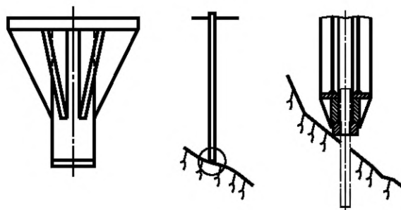
д) Скальный башмак для наклонных скальных поверхностей
