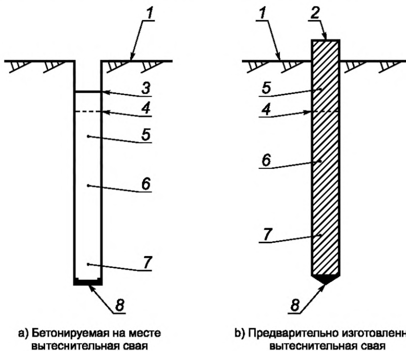
1 — проектная отметка поверхности грунта; 2 — верх сваи; 3 — уровень заливки; 4 — уровень обрезки (уровень отделки); 5 — головная часть сваи; 6 — ствол сваи; 7 — нижняя часть сваи; 8 — пята (башмак) сваи
