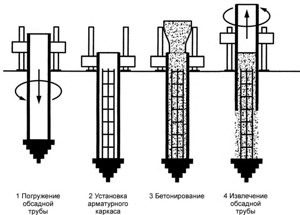
а) Этапы выполнения винтовой набивной вытеснительной сваи с оставаемым наконечником
