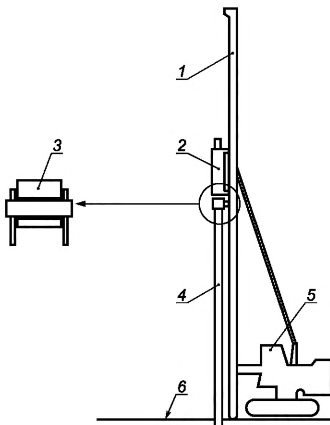
1 — направляющая; 2 — ударный молот; 3 — конструкция наголовника с упругими прокладками; 4 — свая; 5 — основной механизм; 6 — рабочий уровень поверхности грунта
