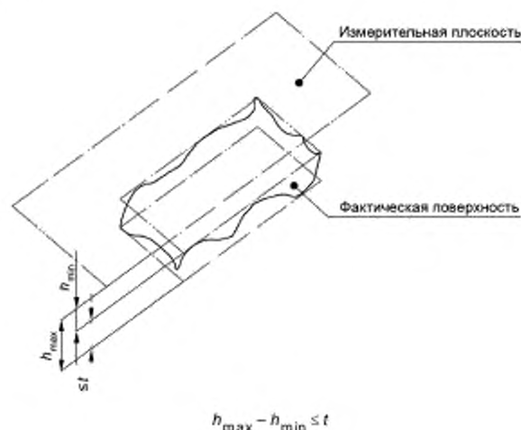
Рисунок 7 — Испытание на плоскостность
