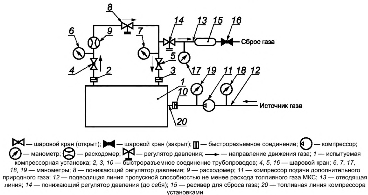
Рисунок А.1 — Типовая схема испытательного стенда
