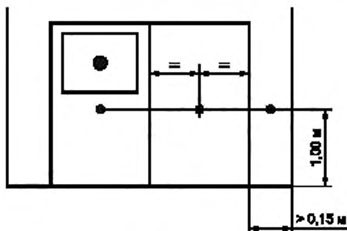
г — Полностью собранная дверь шахты со створками двери и боковыми рамами (пример соответствует рисункам а и б)
