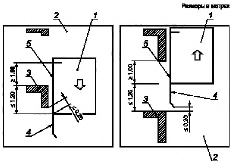
1 — кабина; 2 — шахта; 3 — эстажная площадка; 4 — фартук кабины; 5 — вход в кабину
