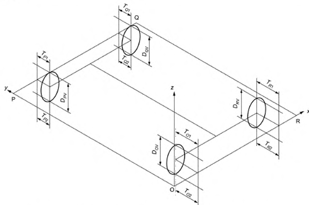
Рисунок 3 — Измерения отклонений положения колес от вертикальной плоскости
