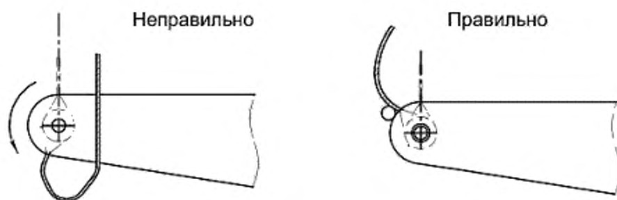
Рисунок 8 – Устройства, исключающие образование петель и перекруток
