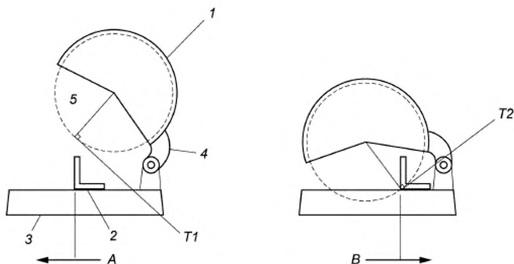
а) Режущая головка в нерабочем положении и в самом нижнем положении
