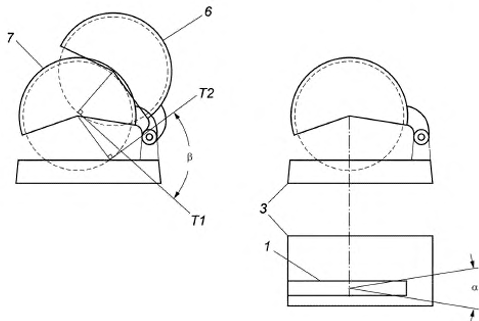
б) Углы отклонения искр
