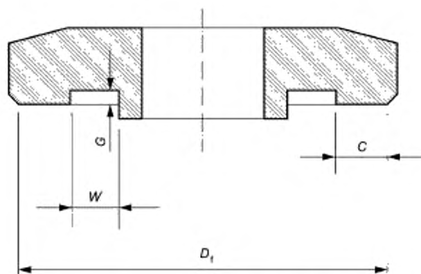
а) конструкция фланца, пример а)
