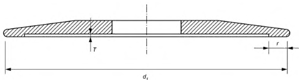
Рисунок 105 — Размеры фланца
