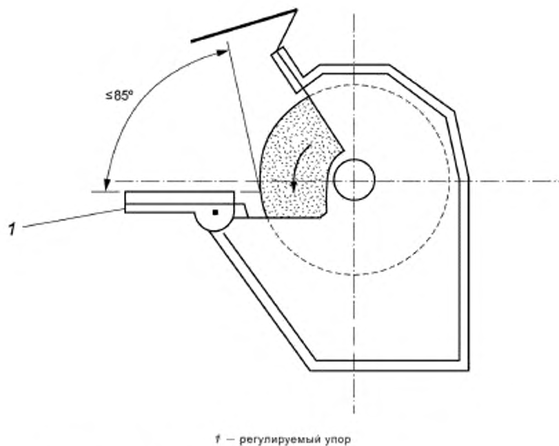
Рисунок 104 — Шлифовально-заточная машина с регулируемым упором
